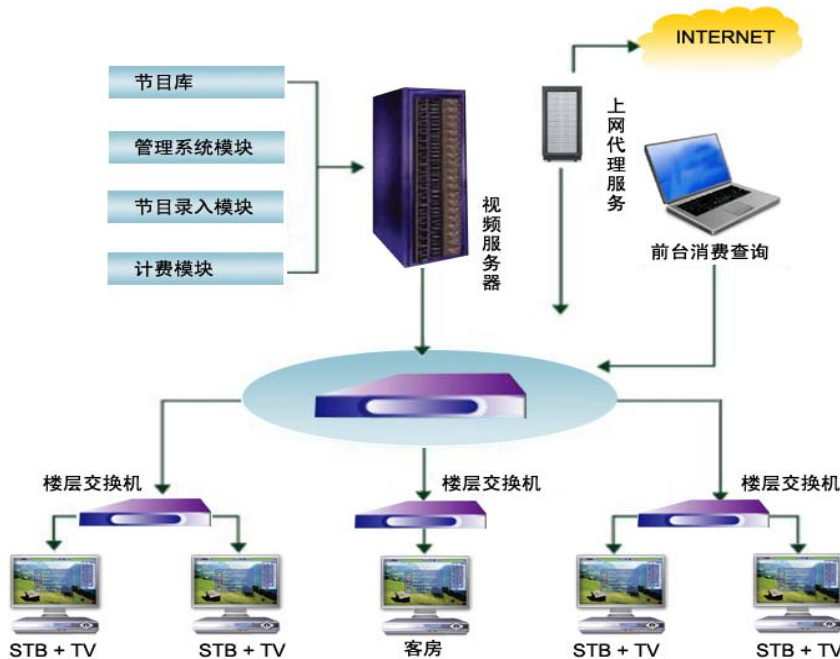
酒店综合信息系统结构图：
